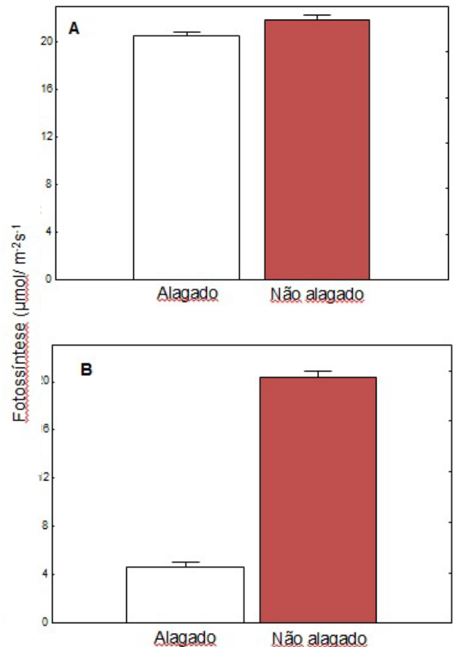
Figura 5. Fotossíntese líquida de folhas do híbrido BRS Ipyporã, um (A) e cinco (B) dias após o início do alagamento do solo.
